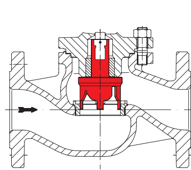
Штицевой затвор с направляющей стержня затвора и посадочного кольца
